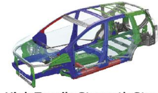
High Tensile Strength Steel ■ 980 MPa class ■ 590 MPa class ■ 440 MPa class
